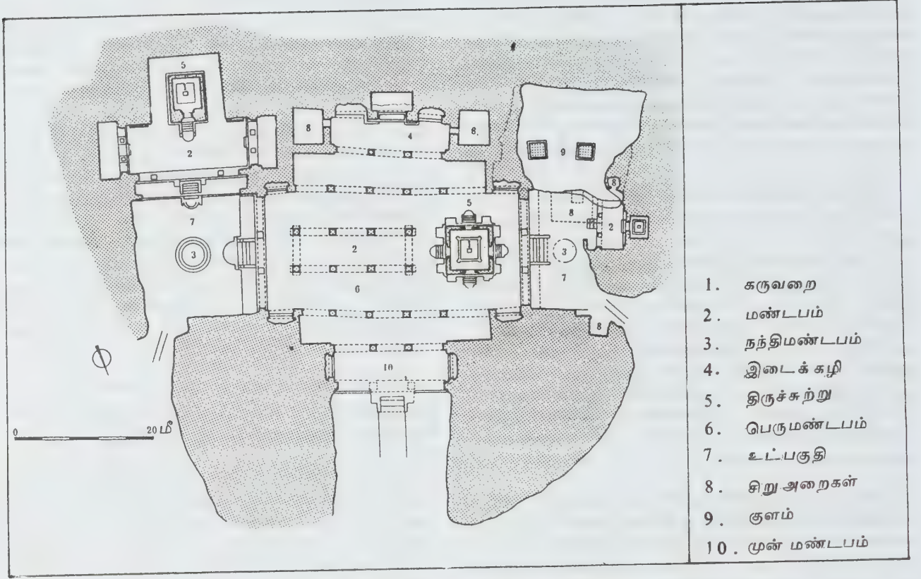
எலிபெண்டாக் குடைவரைகளின் தரைப்படம்
