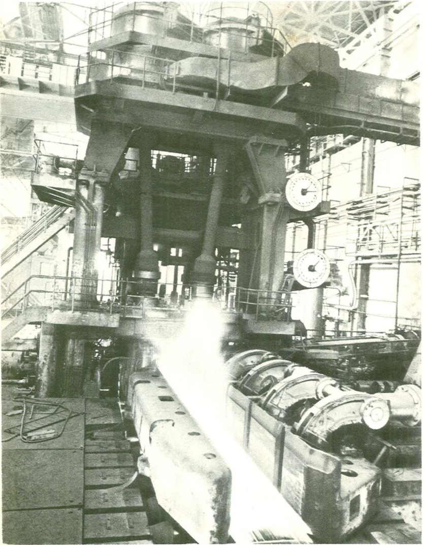
பொக்காரோ உலோகத் தொழிற்சாலை
