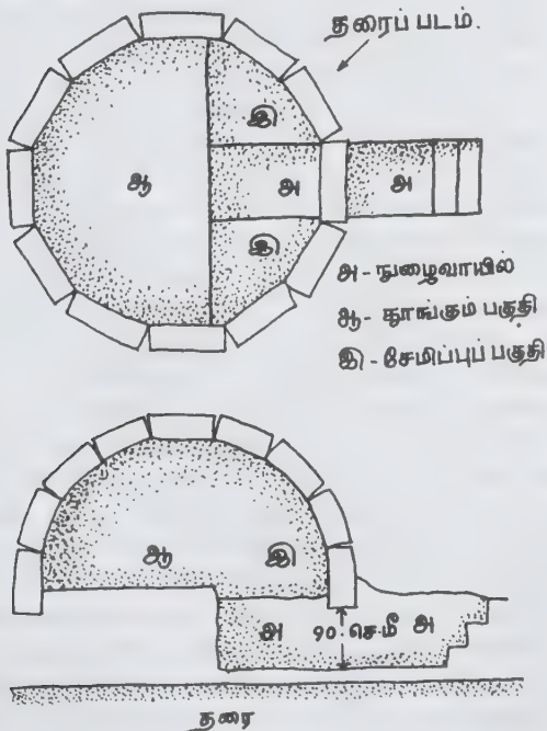
இக்லூவின் அமைப்பு
